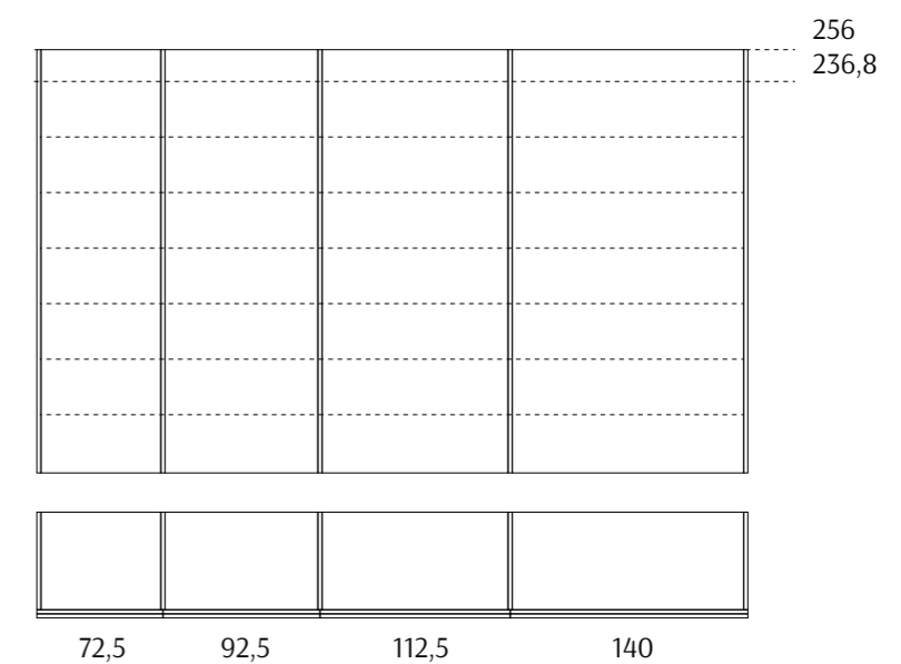
MODULARITÀ ARMADIO ANTE SCORREVOLI E COMPLANARI SLIDING AND COPLANAR DOORS WARDROBE MODULARITY
